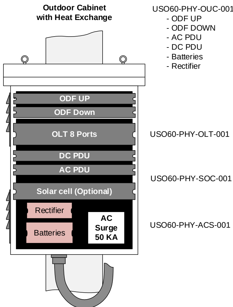
ภาพที่ 1 การติดตั้งอุปกรณ์ภายในชุด Internet Node (OLT)
