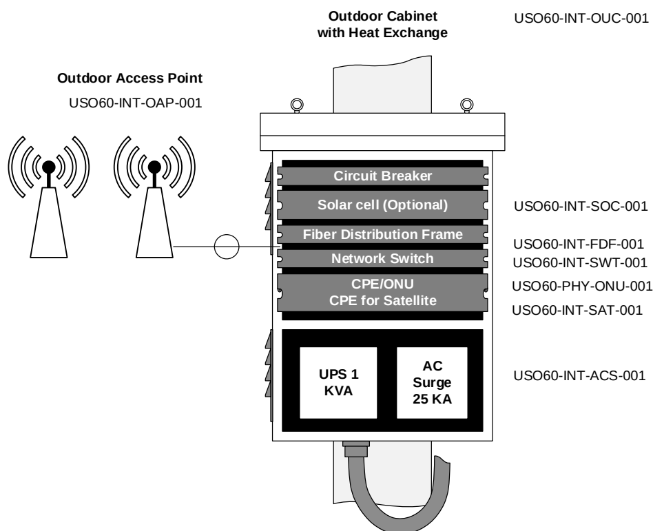
ภาพที่ 7 การติดตั้งชุดตู้ WiFi
