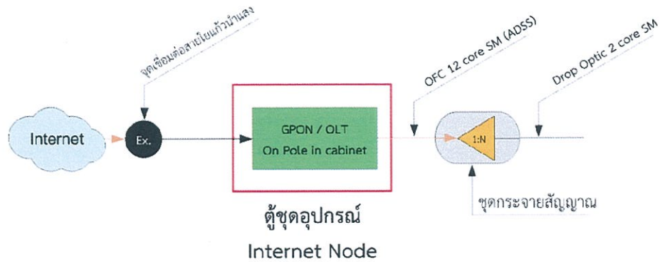
ภาพที่ 3 การติดตั้งและเชื่อมต่อสัญญาณผ่านโครงข่ายภาคพื้นดิน ในจุดติดตั้งที่มีไฟฟ้า
