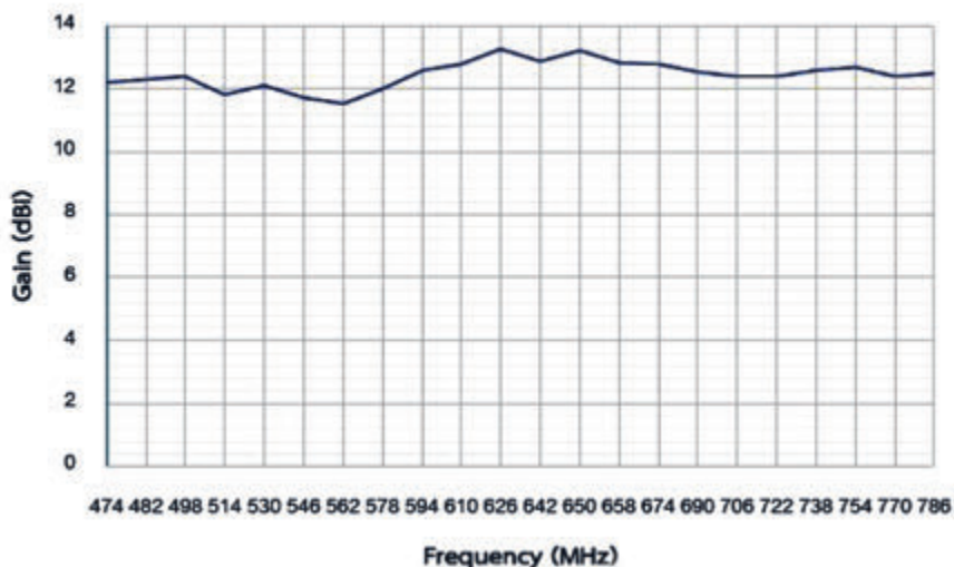
รูปที่ 11 แสดงกราฟค่าอัตราขยายของสายอากาศที่มีคุณสมบัติด้านอัตราขยายที่ดี มีค่าใกล้เคียงกันตลอดช่วงความถี่ใช้งานตั้งแต่ 510 – 790 MHz (ช่องความถี่ 26 – 60)
