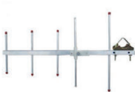
รูปที่ 12 แสดงภาพสายอากาศชนิดมีทิศทางแบบยาگی-อูตะ หรือที่นิยมเรียกว่า “เสาแบบก้างปลา”
