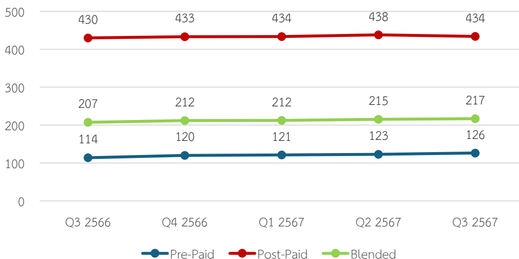
แผนภาพที่ 2.4 รายรับเฉลี่ยต่อเดือนต่อเลขหมายของบริการโทรศัพท์เคลื่อนที่ภายในประเทศ (บาท)
