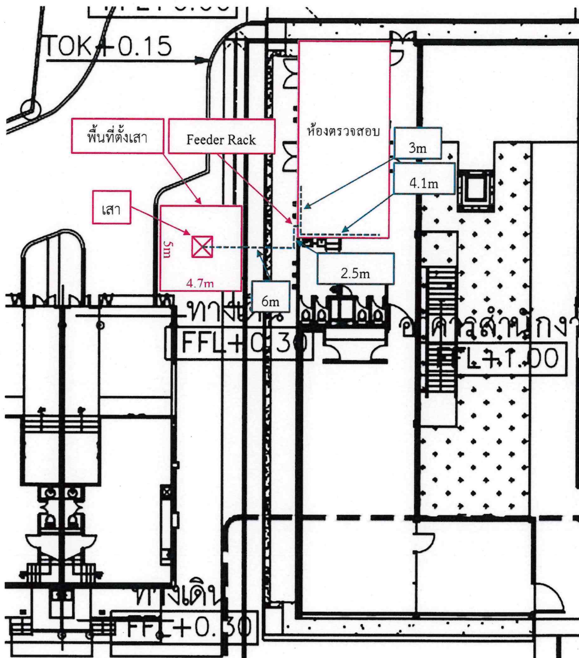
แนวการติดตั้งรางเดินสายนำสัญญาณ (Feeder Rack) จากตัวเสาไปยังห้องตรวจสอบ
