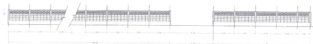
Section A-A
