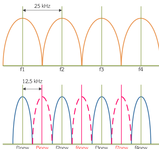
ช่องความถี่ภายหลัง Narrowbanding - เส้นทึบ แสดงช่องความถี่ที่ได้ปรับลด channel spacing แล้ว - เส้นประ แสดงช่องความถี่ที่เกิดขึ้นใหม่
